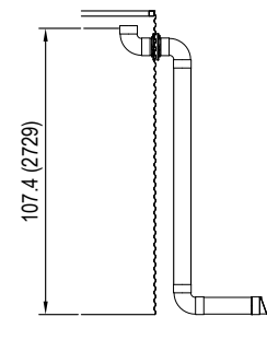
OVERFLOW SCALE: 1:50
