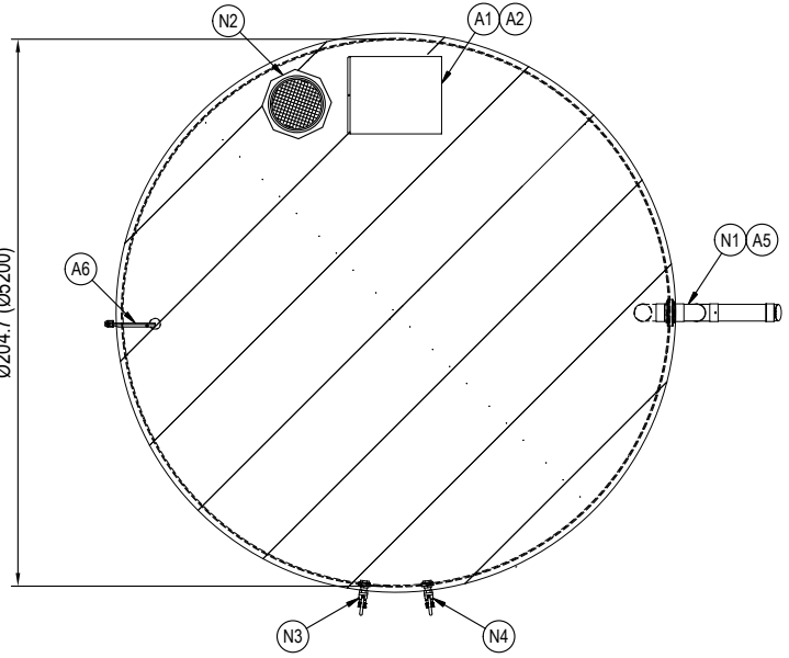
TANK PLAN SCALE: 1:50
