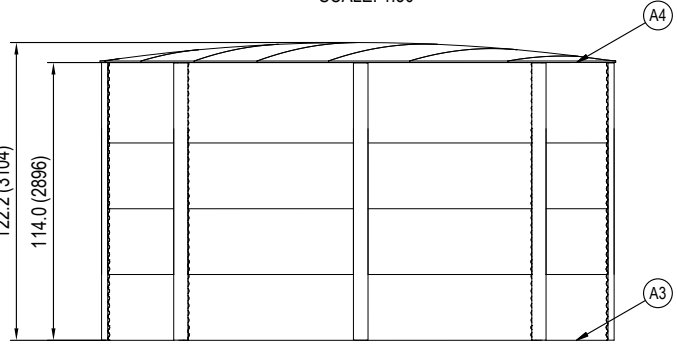
TANK ELEVATION SCALE: 1:50
