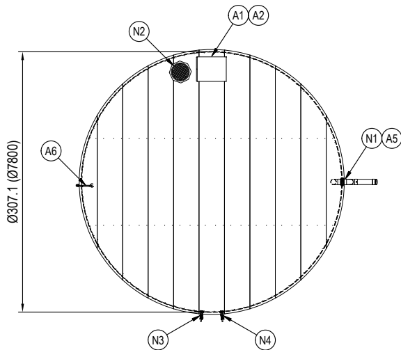
TANK PLAN SCALE: 1:100
