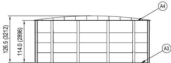
TANK ELEVATION SCALE: 1:100
