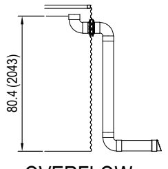
OVERFLOW SCALE: 1:50
