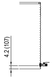
OUTLET SCALE: 1:50
