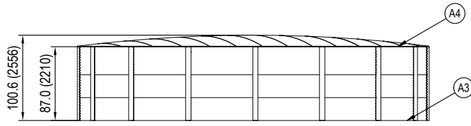
TANK ELEVATION SCALE: 1:100
