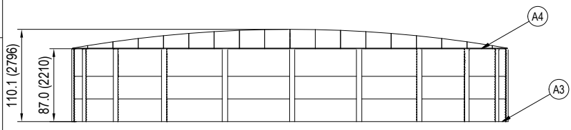
TANK ELEVATION SCALE: 1:100
